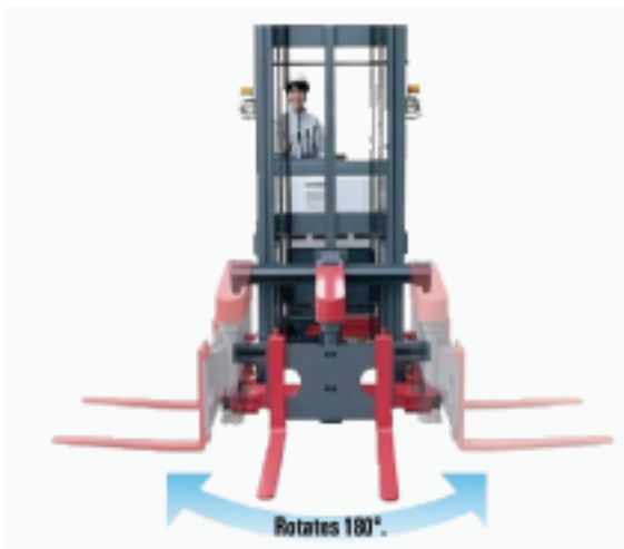
采用意大利ZAPI AC控制器,全液助力转向,通过多路阀轻松控制旋转头左右180度旋转。
